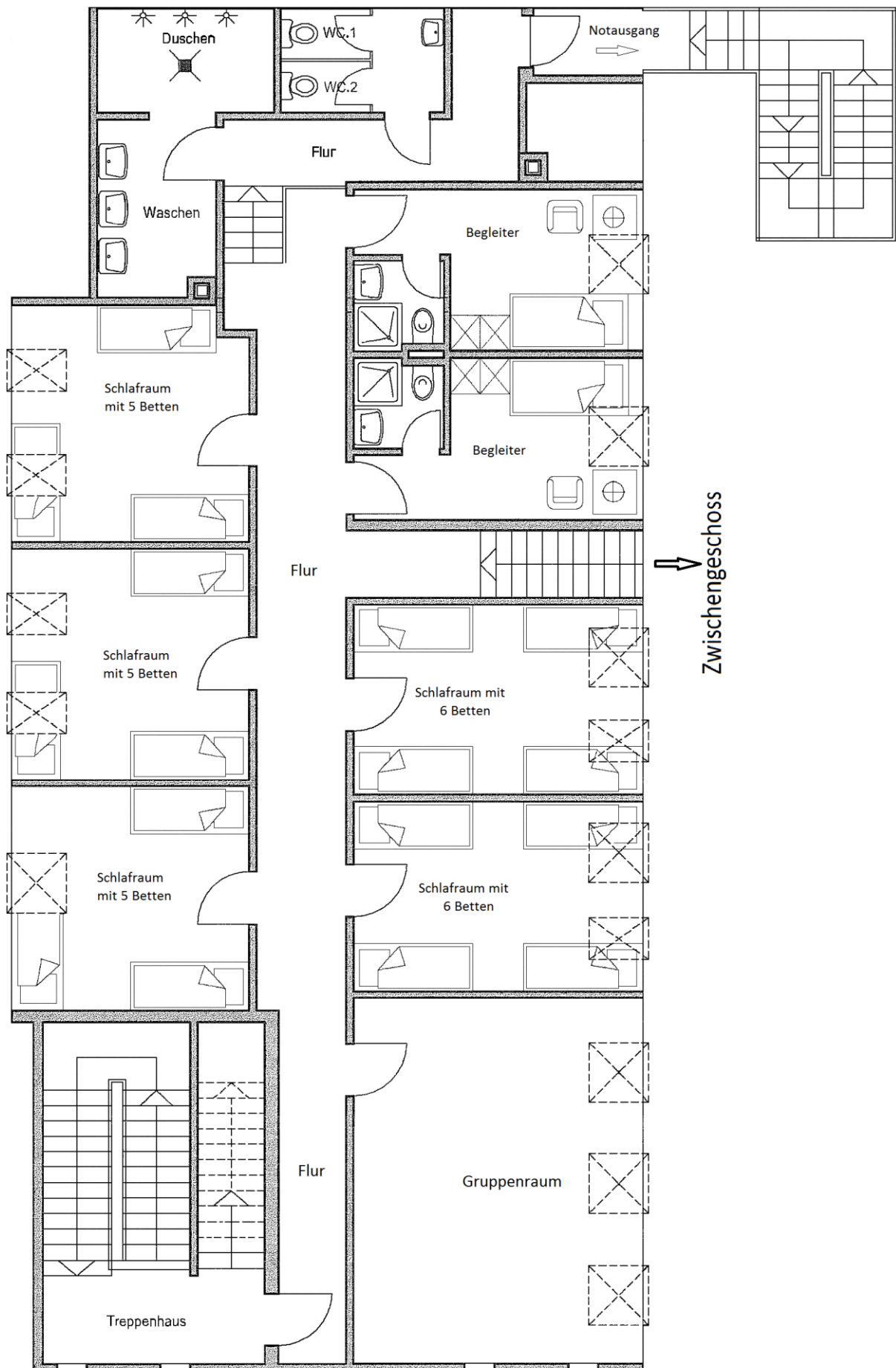
1. Geschoss
